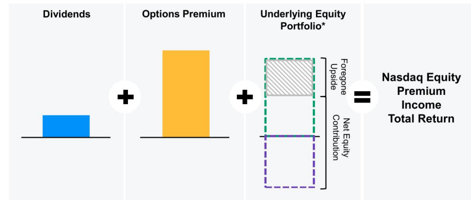
图：JEPQ产品收益构成
